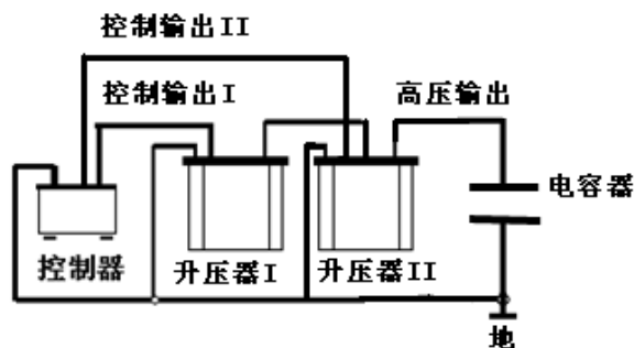
图 11 测量电容器的连线图
