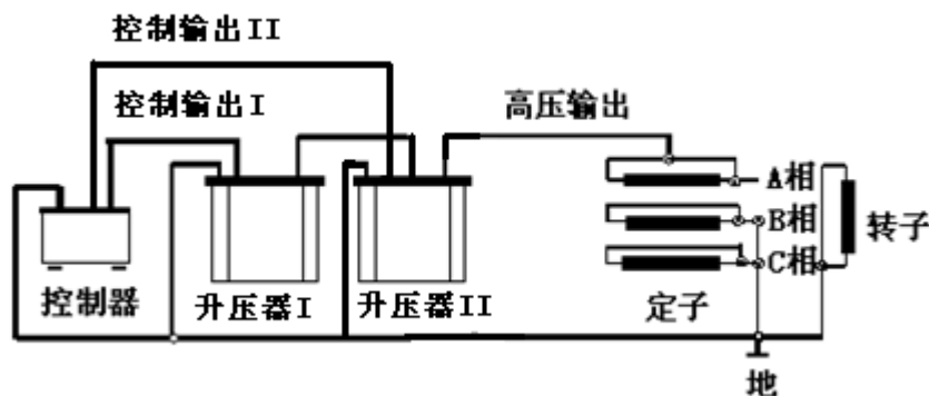
图 10 测量定子的某相连线图
