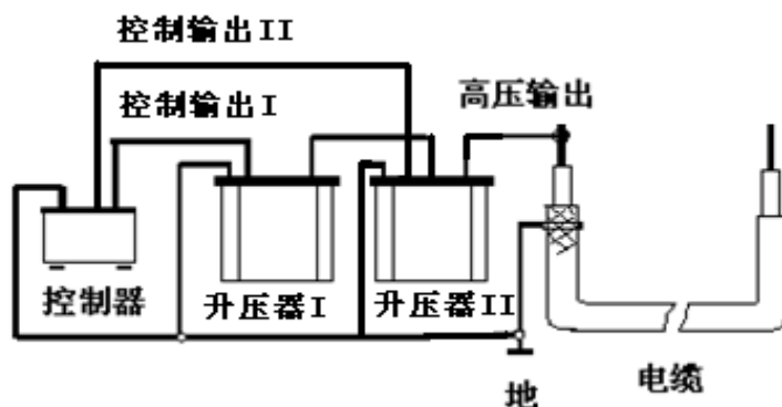
图 9 单相测量连线图
