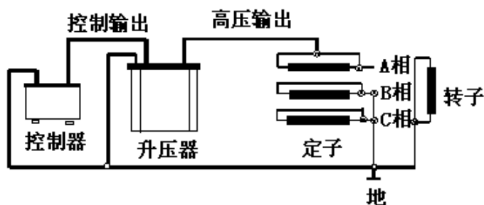
图 8 测量定子的某相连线图
