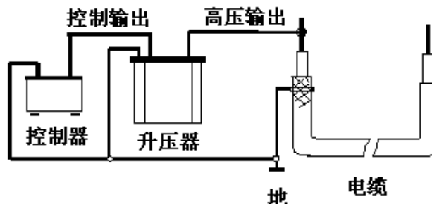
图 7 单相测量连线图
