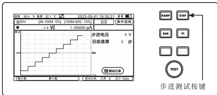
图 9 （步进 SIEP 测量）
