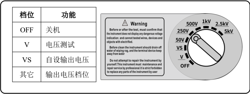
图 2 （旋钮档位图）
