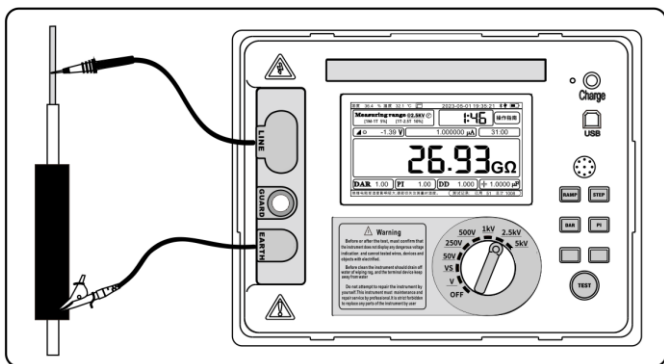
图 16（接常规两线测量接线方式）
