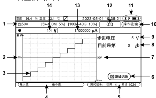
图6（步进 STEP 测量模式界面）
