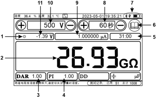
图 5 （自设输出电压测量模式界
