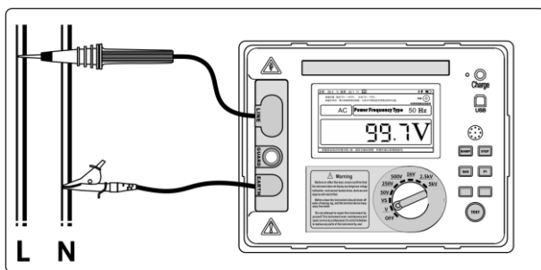
图 10（电压接线示意图）
