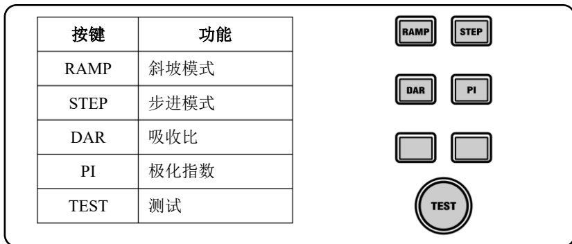
图 3 （按钮图）
