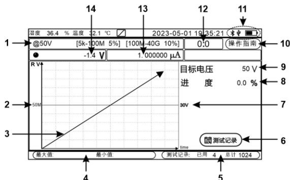
图 7 （斜坡 RAMP 测量模式界面）
