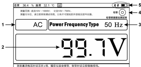
图 11（电压测试界面）
