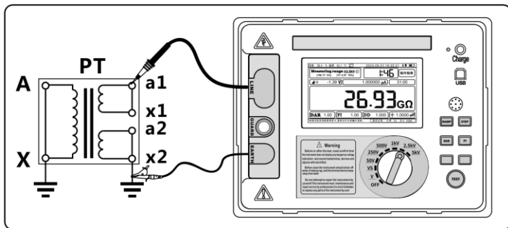
图 22 (二次绕组间绝缘电阻测试)
