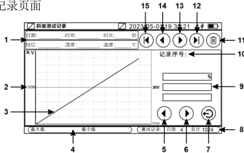
图 14（斜坡测试记录界面）
