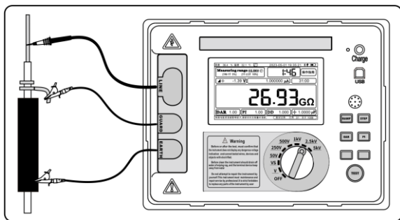
图 17（超高阻值三线测量接线方式）
