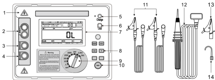
图 1（仪表结构图）
