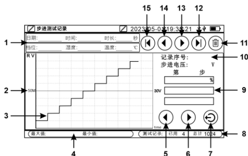
图 15（步进测试记录界面）
