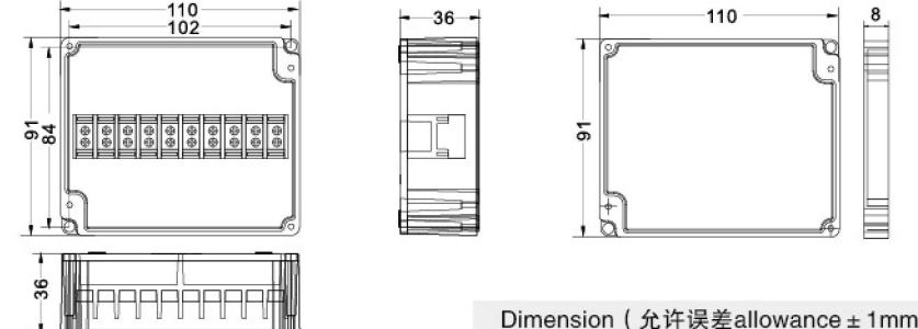
型号 (Model) : ZX-AG-10P-M 尺寸 (Size) : 91×110×43mm
