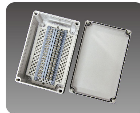
型号 (Model) : ZX-AG-40P-S 尺寸 (Size) : 150 × 250 × 100mm
