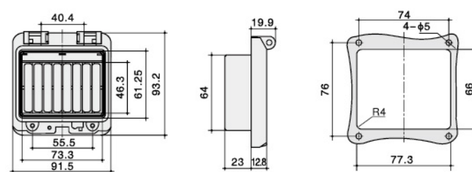
型号 (Model) : ZX-4
