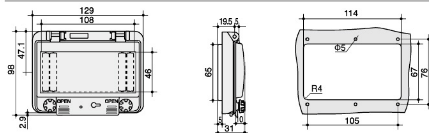
型号 (Model) : ZX-6B
