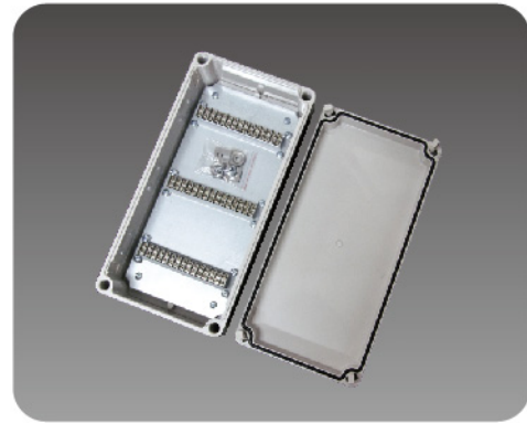
型号 (Model) : ZX-AG-45P 尺寸 (Size) : 380 × 190 × 100mm
