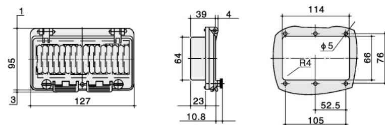
型号 (Model) : ZX-6
