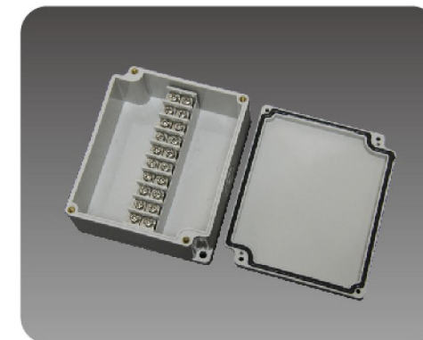
型号 (Model) : ZX-AG-10P-M 尺寸 (Size) : 91×110×43mm
