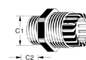
C Body 基本幅体
