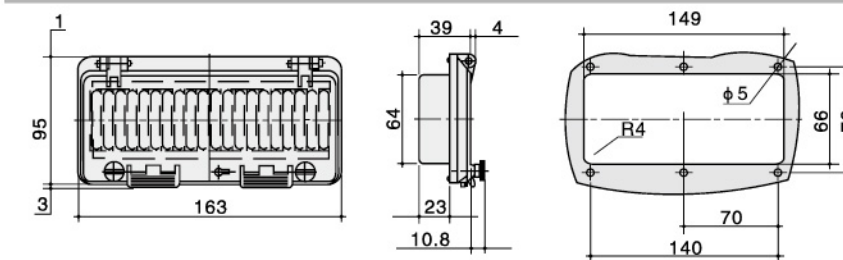
型号 (Model) : ZX-8
