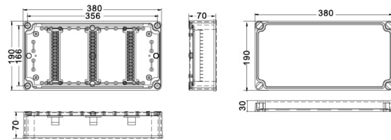
型号 (Model) : ZX-AG-45P 尺寸 (Size) : 380 × 190 × 100mm
