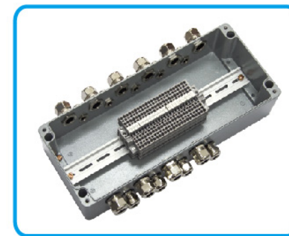
▲ 配接线端子 With terminal block
