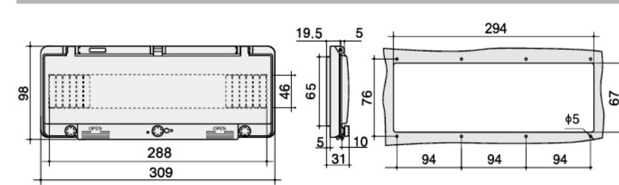
型号 (Model) : ZX-16A
