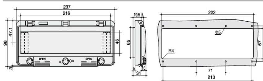
型号 (Model) : ZX-12B
