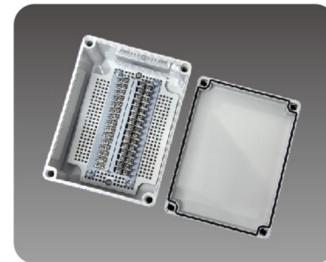
型号 (Model) : ZX-AG-30P-S 尺寸 (Size) : 150 × 200 × 100mm
