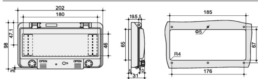
型号 (Model) : ZX-10B
