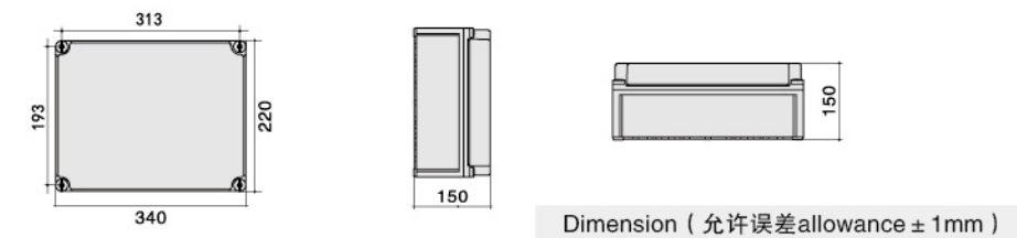
型号 (Model) : ZX-PCS-223415 尺寸 (Size) : 220 × 340 × 150mm
