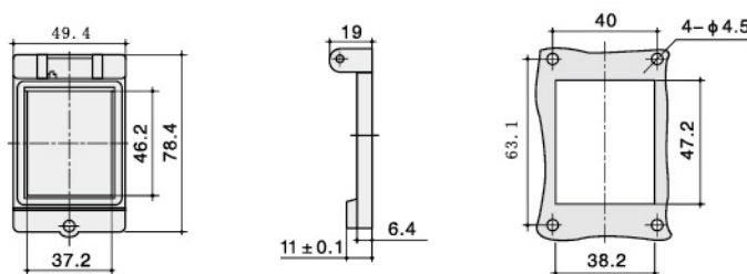
型号 (Model) : ZX-2
