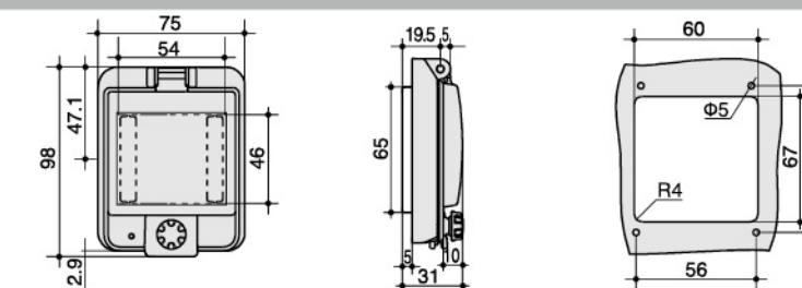
型号 (Model) : ZX-3B
