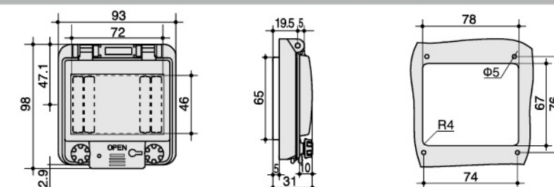
型号 (Model) : ZX-4B
