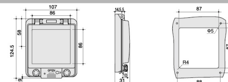
型号 (Model) : ZX-5B
