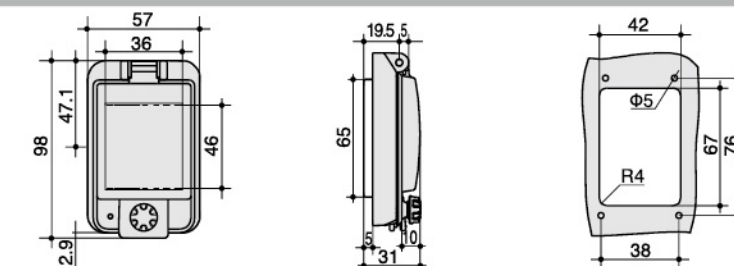
型号 (Model) : ZX-2B
