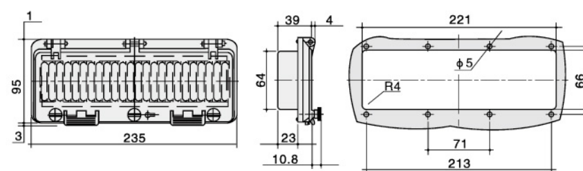
型号 (Model) : ZX-12
