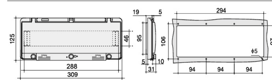
型号 (Model) : ZX-16B
