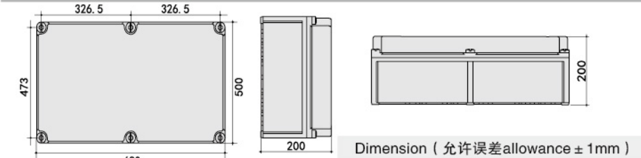
型号 (Model) : ZX-PCS-506820 尺寸 (Size) : 500 × 680 × 200mm
