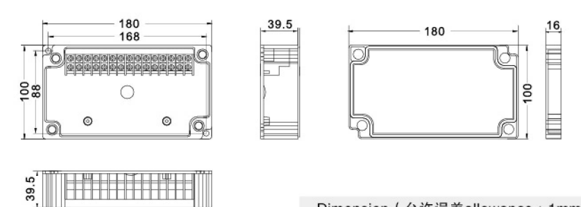
型号 (Model) : ZX-AG-15P 尺寸 (Size) : 100×180×55mm
