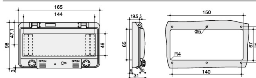
型号 (Model) : ZX-8B
