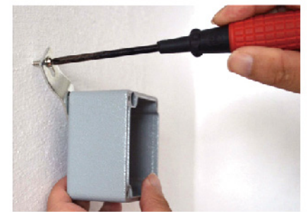
通过安装挂脚固定
