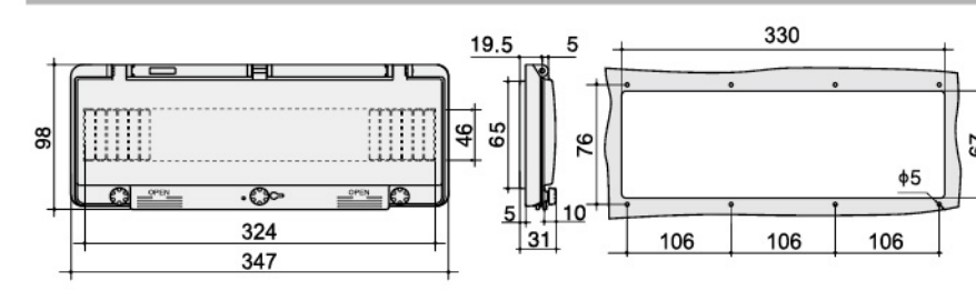
型号 (Model) : ZX-18B
