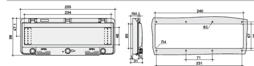
型号 (Model) : ZX-13B
