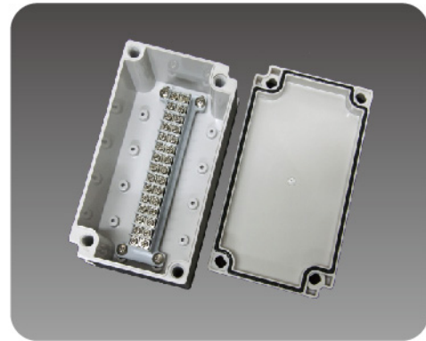
型号 (Model) : ZX-AG-15P-M 尺寸 (Size) : 100 × 180 × 75mm
