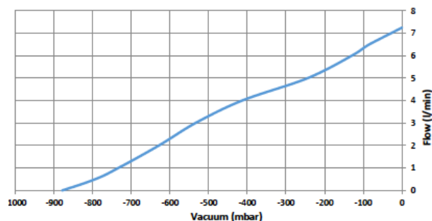
真空/流量曲线
