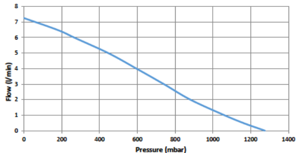
压力流量曲线
