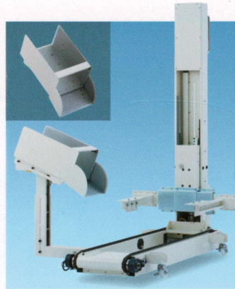
CS-860-2SHA シュータ付き With Chute
