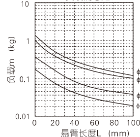
选型曲线图(9) 最大速度≤300(mm/s) 负载偏心距：200mm
