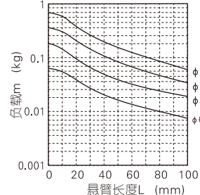
选型曲线图(11) 最大速度≤500(mm/s) 负载偏心距：100mm
