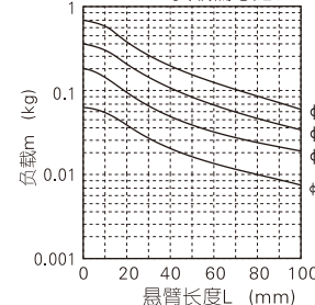
选型曲线图(10) 最大速度≤500(mm/s) 负载偏心距：50mm
