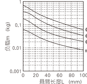
选型曲线图(12) 最大速度≤500(mm/s) 负载偏心距：200mm
