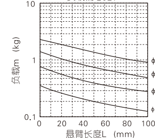
选型曲线图(5) 最大速度≤100(mm/s) 负载偏心距：100mm
