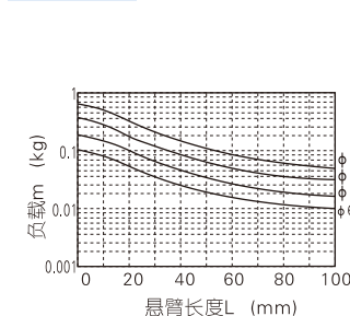
选型曲线图(3) 最大速度≤500(mm/s)
