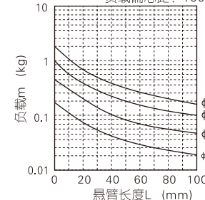
选型曲线图(8) 最大速度≤300(mm/s) 负载偏心距：100mm
