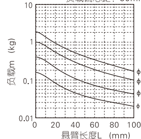
选型曲线图(7) 最大速度≤300(mm/s) 负载偏心距：50mm
