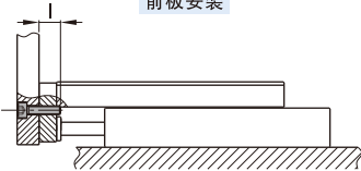
前板安装
