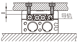
顶板安装
