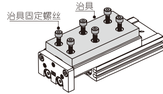
顶板安装
