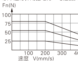
水平运行许用驱动力 F_n 与速度关系曲线
