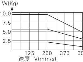
水平运行负载与速度关系曲线
