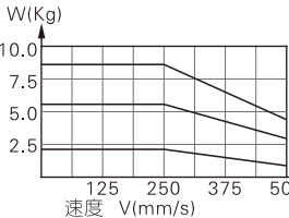
垂直运行负载与速度关系曲线
