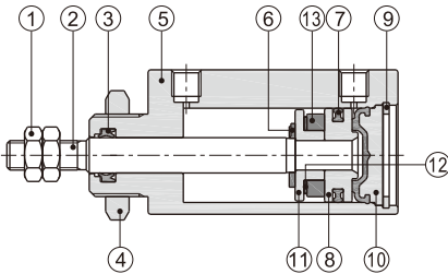
MPG-S(Φ8~Φ16)
