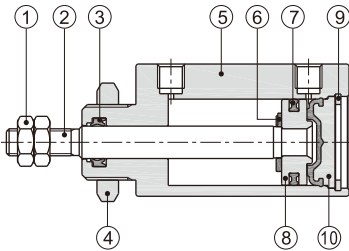
MPG(Φ8~Φ16)
