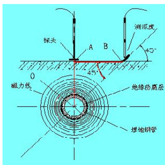
45 度法示意图
