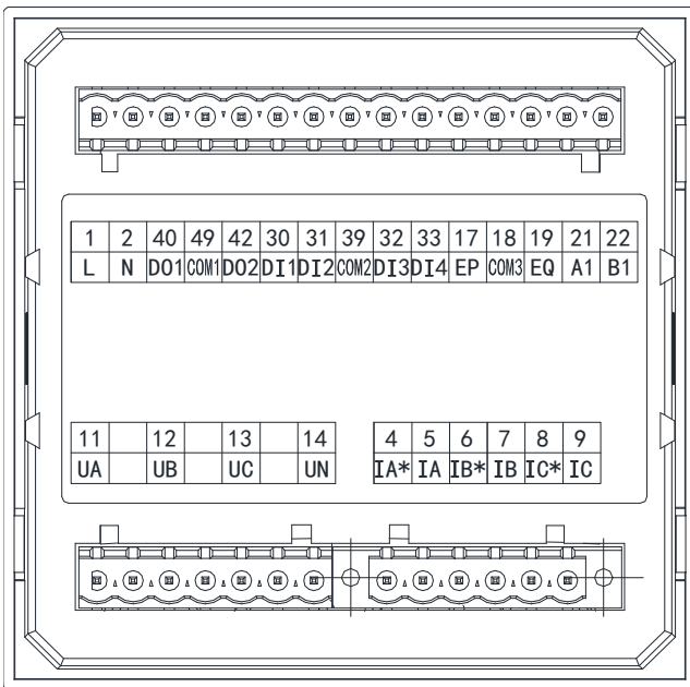
图 13 APM520 基础款接线图
