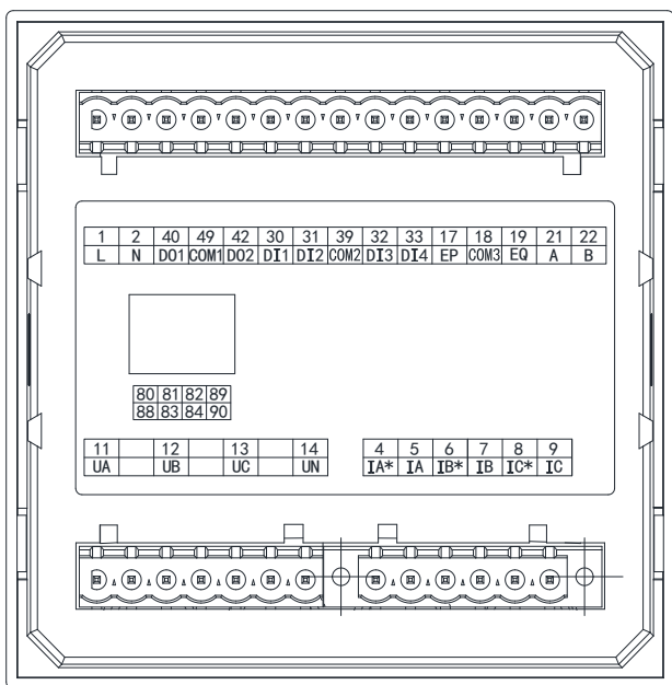
图 15 APM520 扩展测温/漏电接线图
