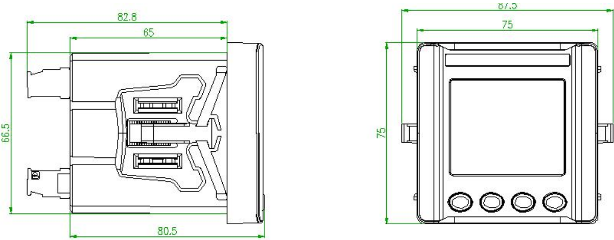
图 2 APM510 尺寸图
