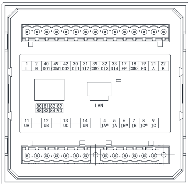
图 17 APM520 扩展 CE 接线图
