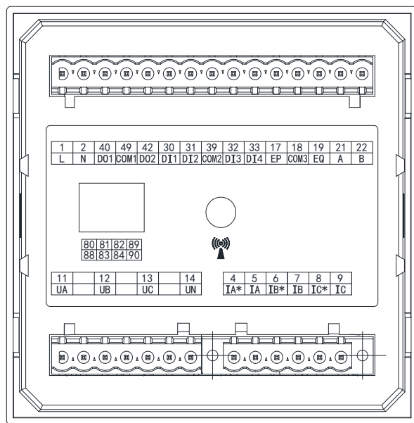
图 18 APM520 扩展 WF/LoRa 接线图
