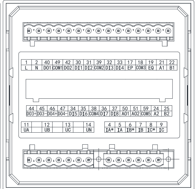
图 14 APM520 扩展 K/2M/2C 接线图
