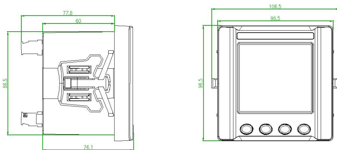
图 3 APM520 尺寸图
