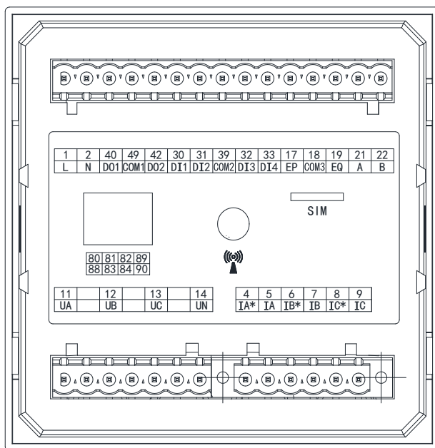
图 16 APM520 扩展 4G/NB 接线图
