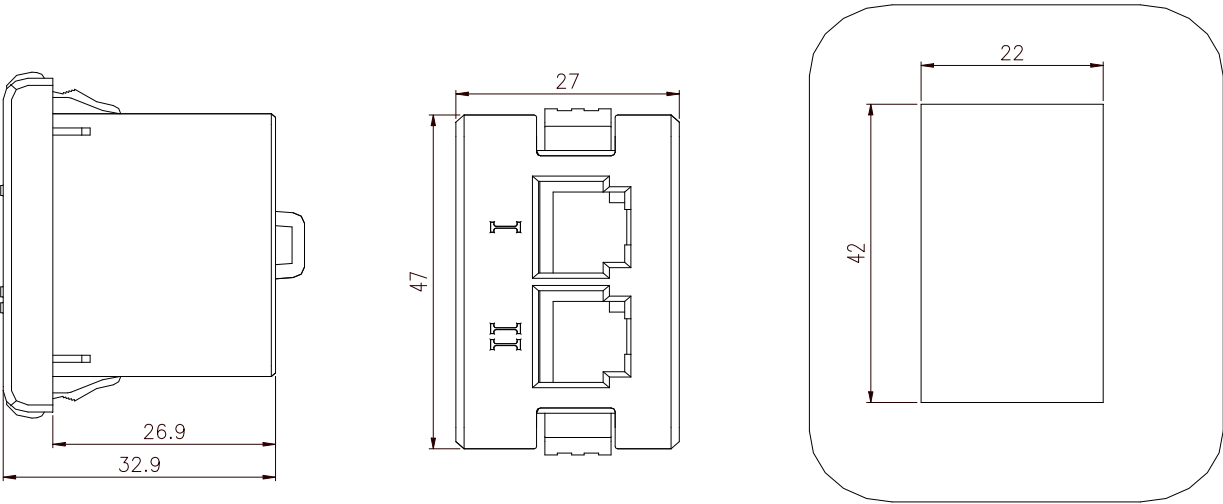
开孔尺寸
