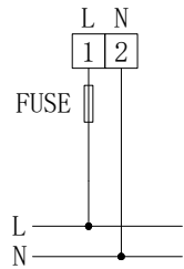
AMB1X0-A(W)-P1 辅助电源
