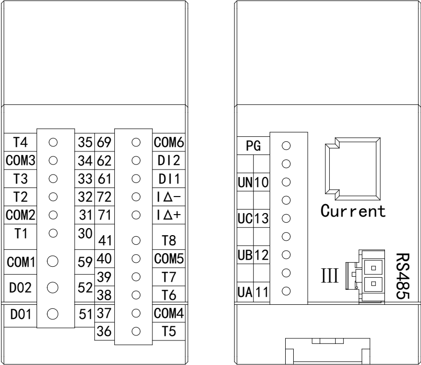
AMB1X0-A(/W)信号取电
