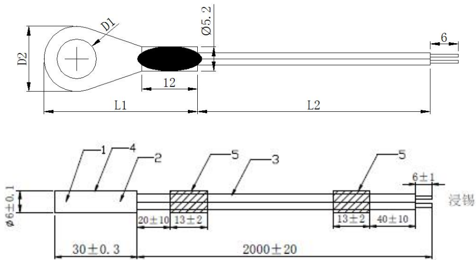
4) 温度传感器（单位：mm）
