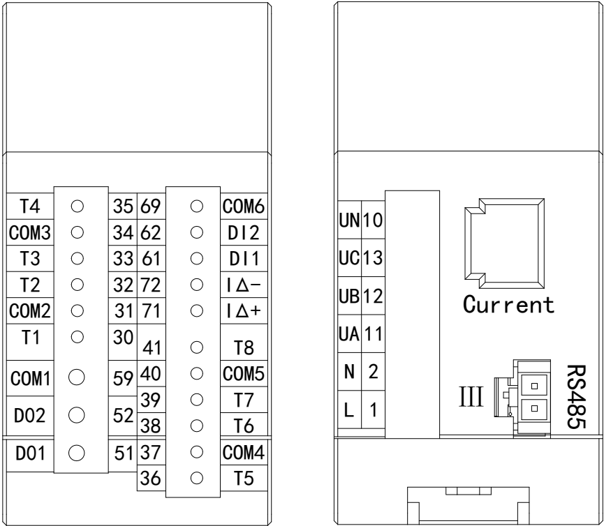
AMB1X0-A(/W)-P1 独立辅助电源
