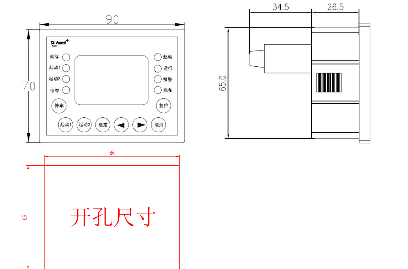
图 12 90L 显示模块外形尺寸
