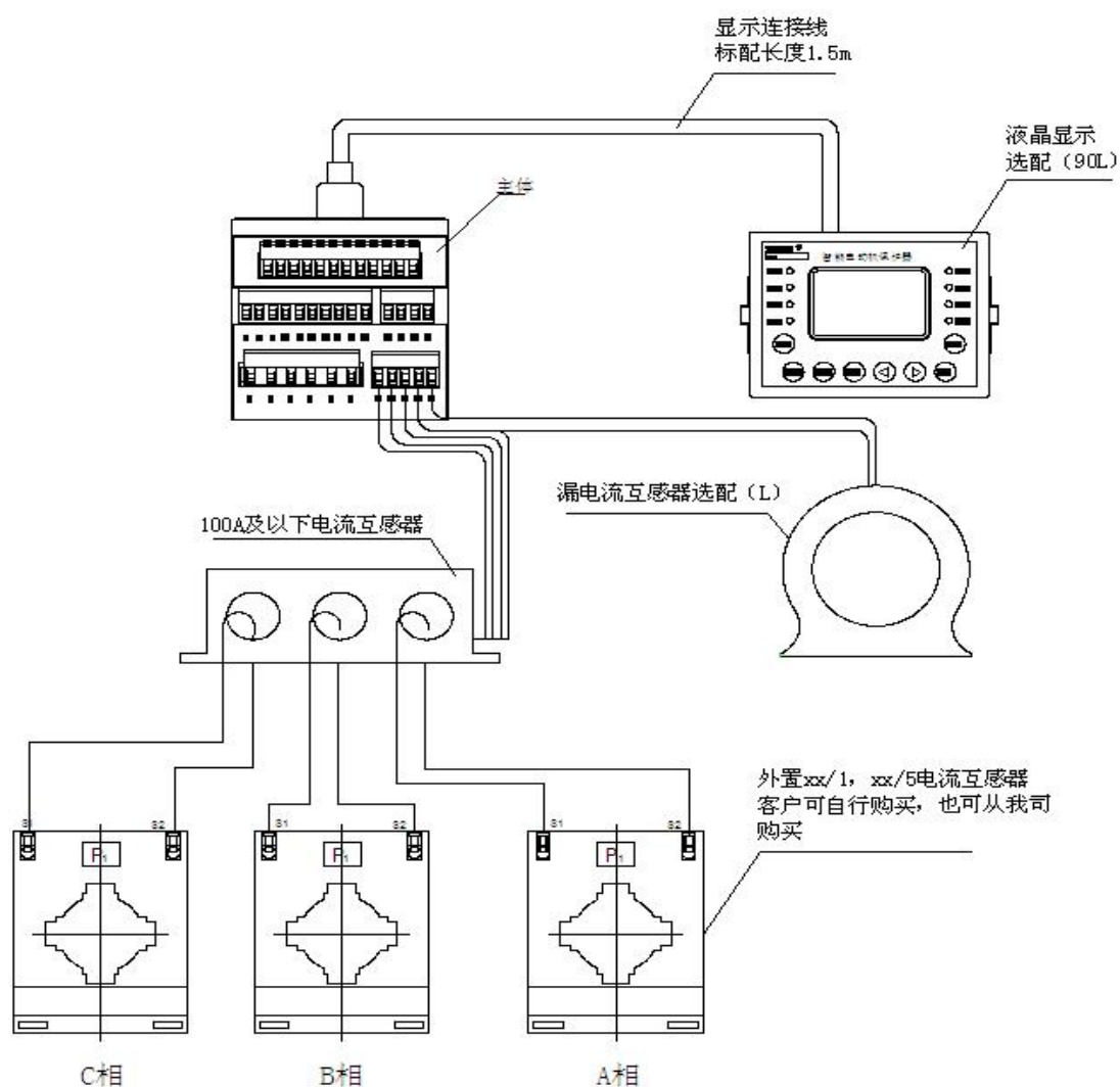
图 5 ARD3-1、ARD3-5 产品组成 (1A 绕线五圈)
