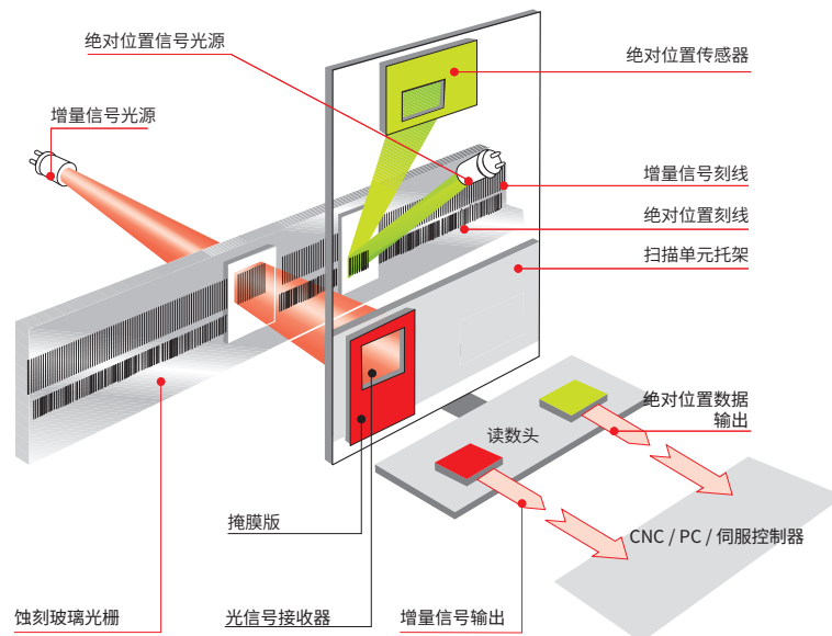
刻线玻璃光栅 (图.1)
