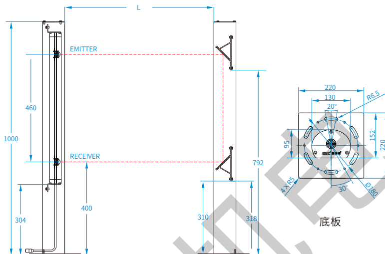
安装尺寸示意图
