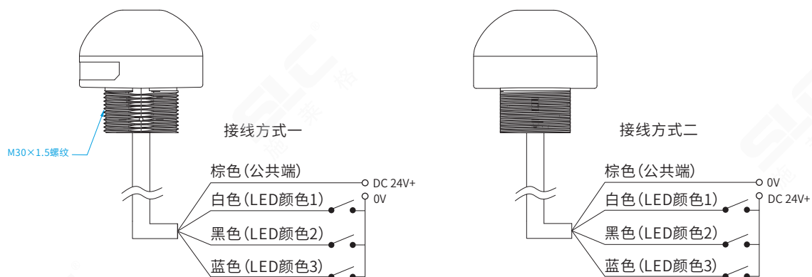
◆ SML50三色灯接线示意图
