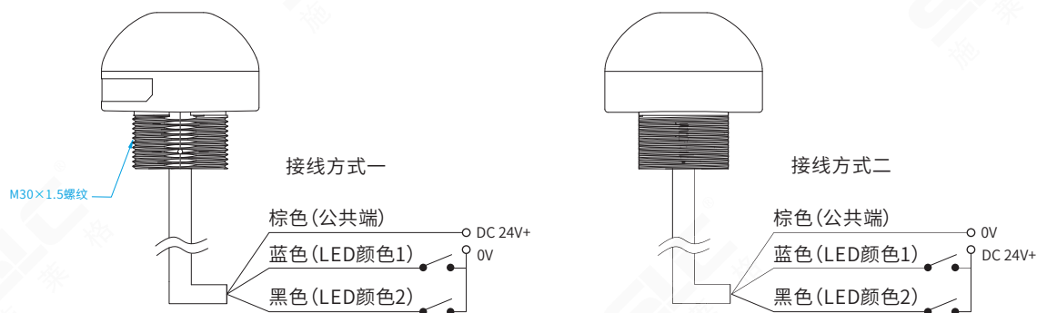
◆ SML50两色灯接线示意图
