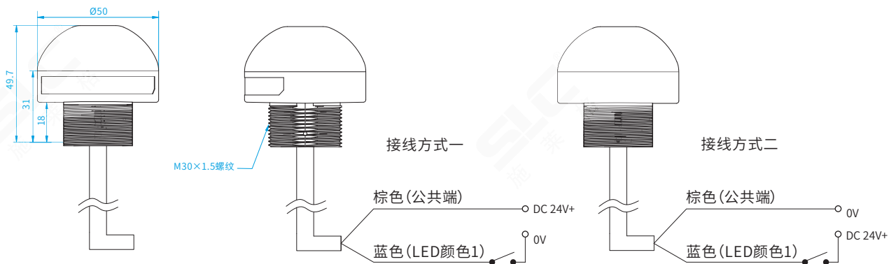
◆ SML50单色灯接线示意图
