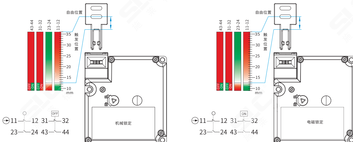
TTS2-K3触头触发行程图
