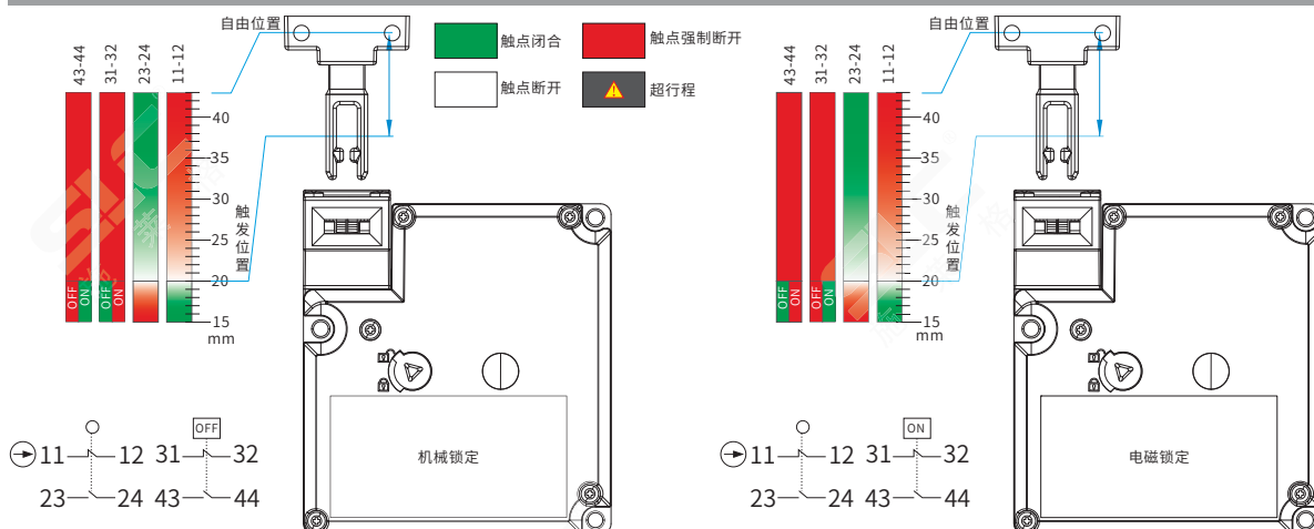
TTS2-K2触头触发行程图
