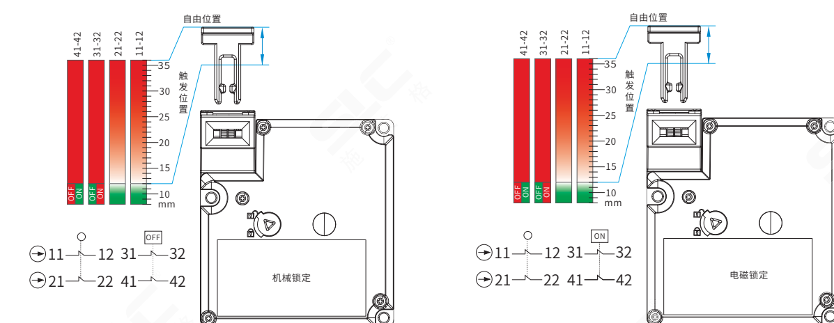
TTS2-K3触头触发行程图
