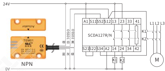
TEM01系列RFID开关双路级联NPN型输出应用接线示例
