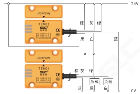
TEM01系列RFID开关双路级联PNP型输出级联接线示例
