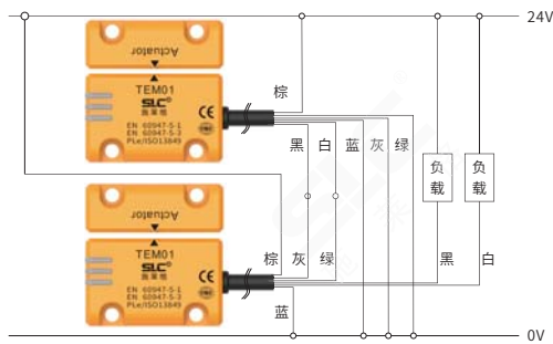
TEM01系列RFID开关双路级联NPN型输出级联接线示例
