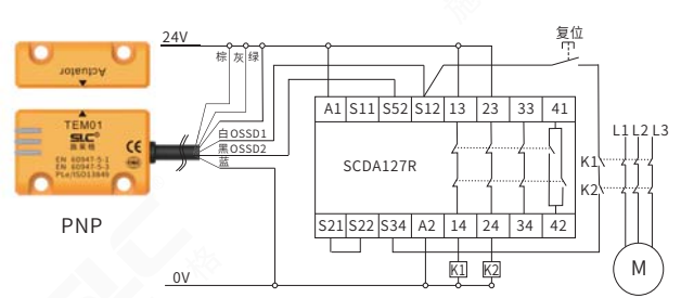
TEM01系列RFID开关双路级联PNP型输出应用接线示例
