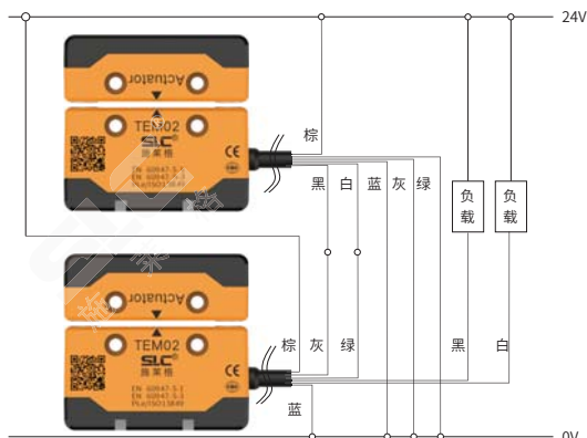
TEM02系列安全开关级联NPN型输出级联接线示例
