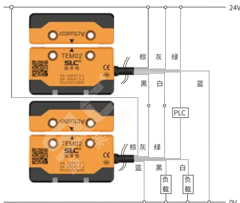
TEM02系列安全开关级联PNP型输出级联接线示例
