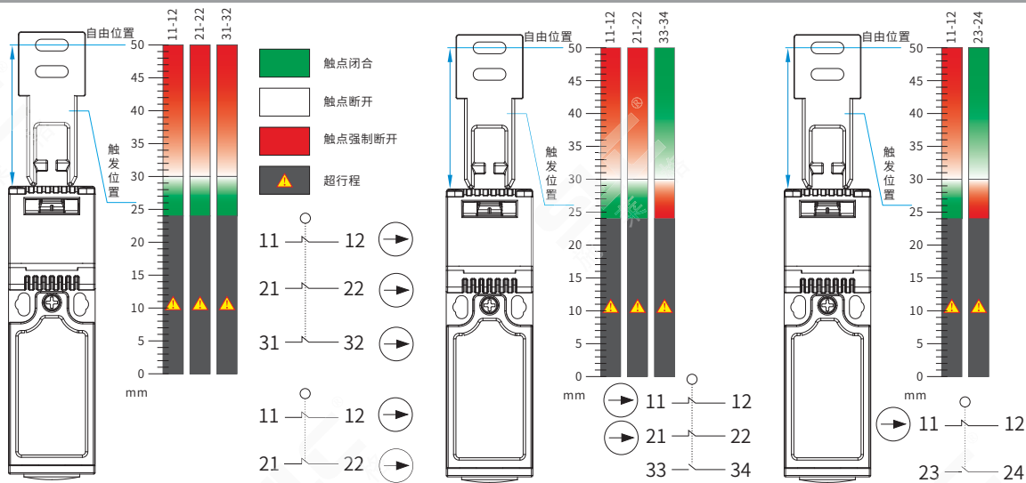
TTS1K1触发触头行程图
