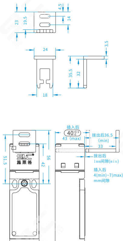
TTS1K1弯钥匙
