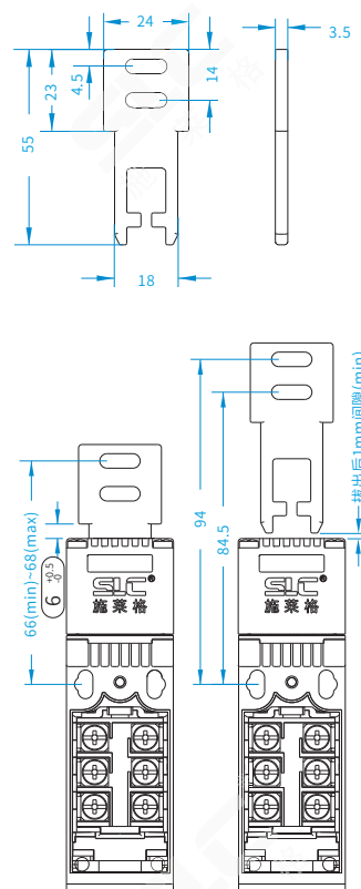
TTS1K2直钥匙
