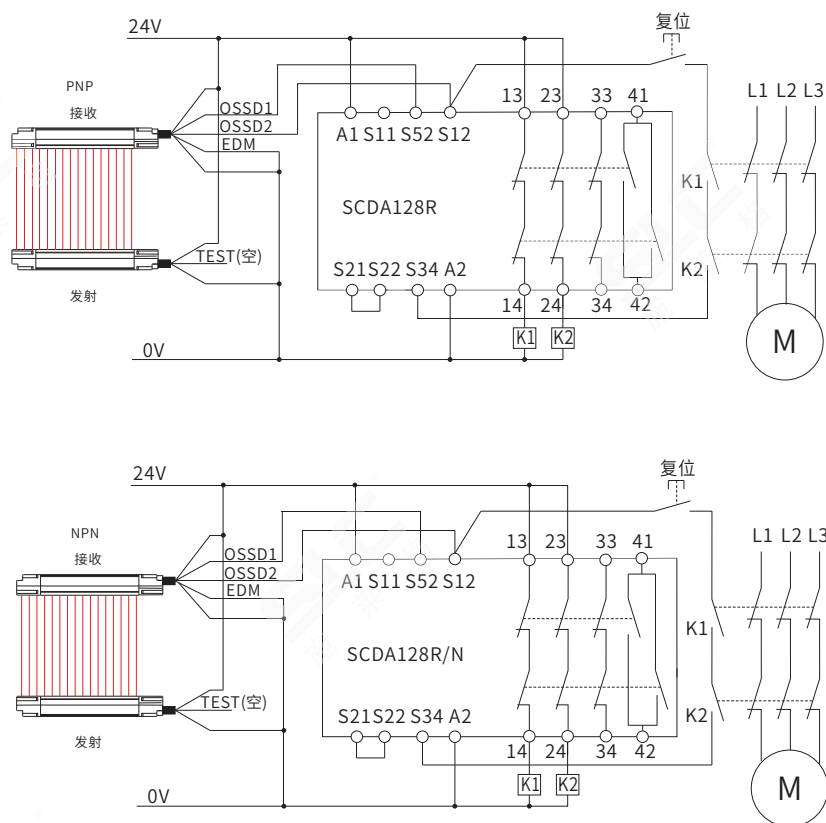
SLC系列光栅，受监视的手动复位，输出监视
