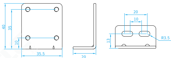
名称: TRL1一号安装支架
