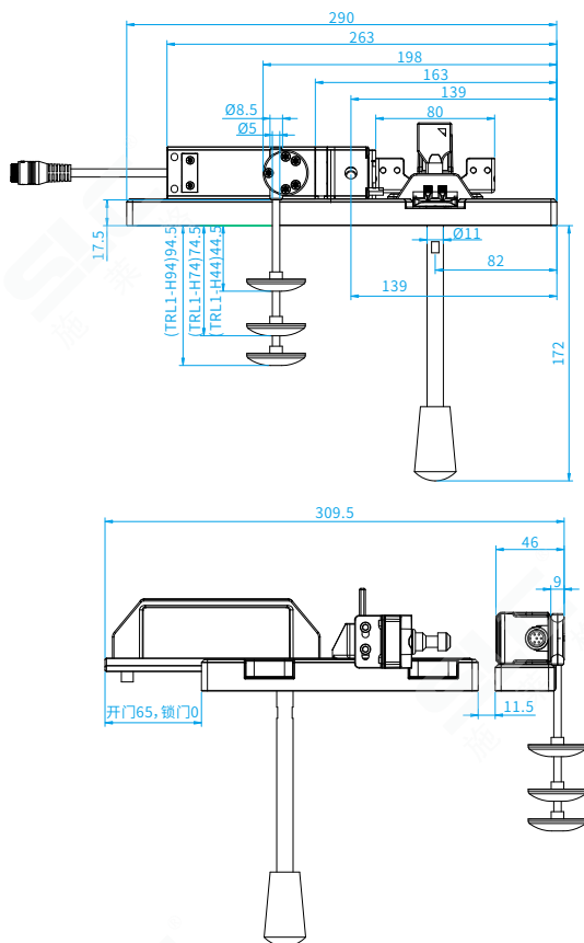
TRL1安全连锁(右开门)安装尺寸
