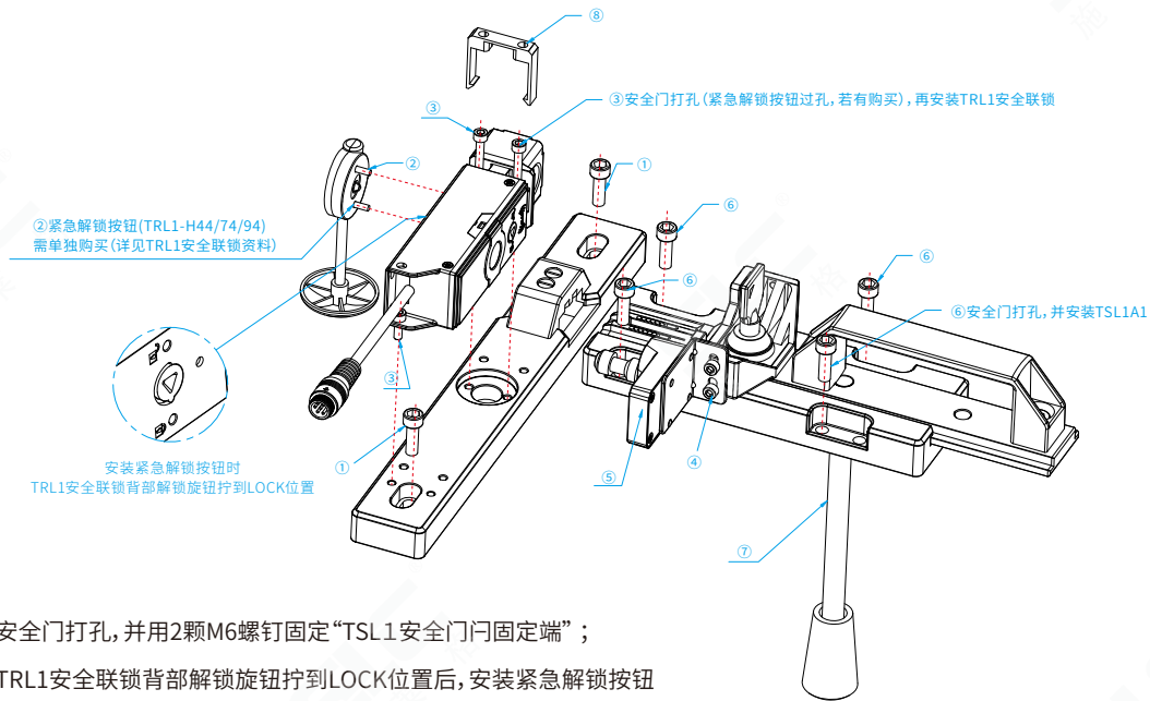
TRL1系列安全联锁安装图
