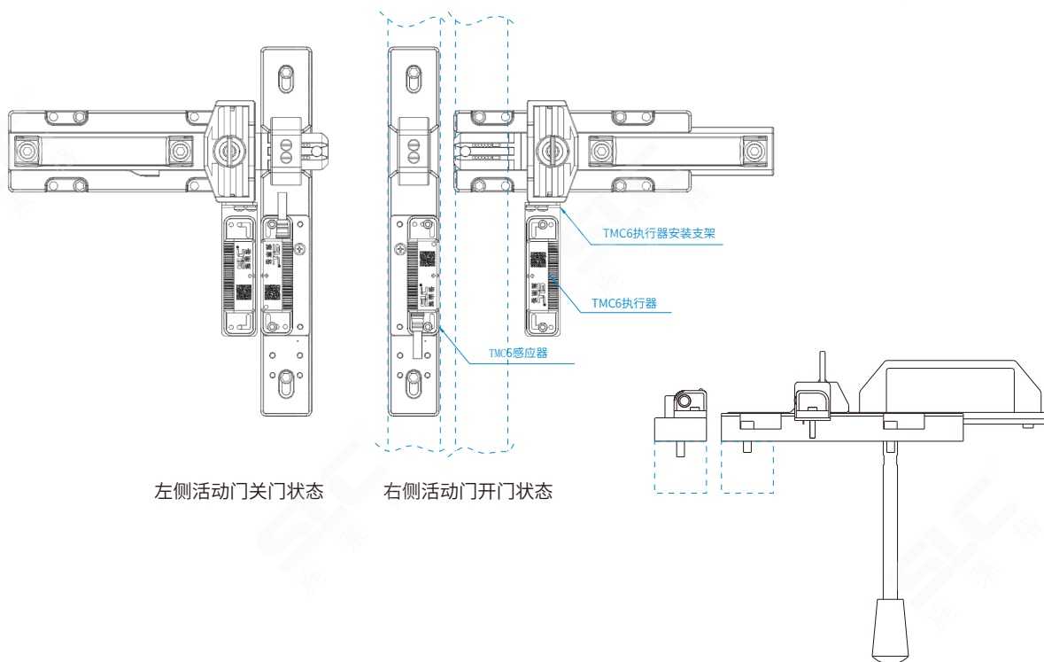
TMC6系列射频RFID安全开关安装图
