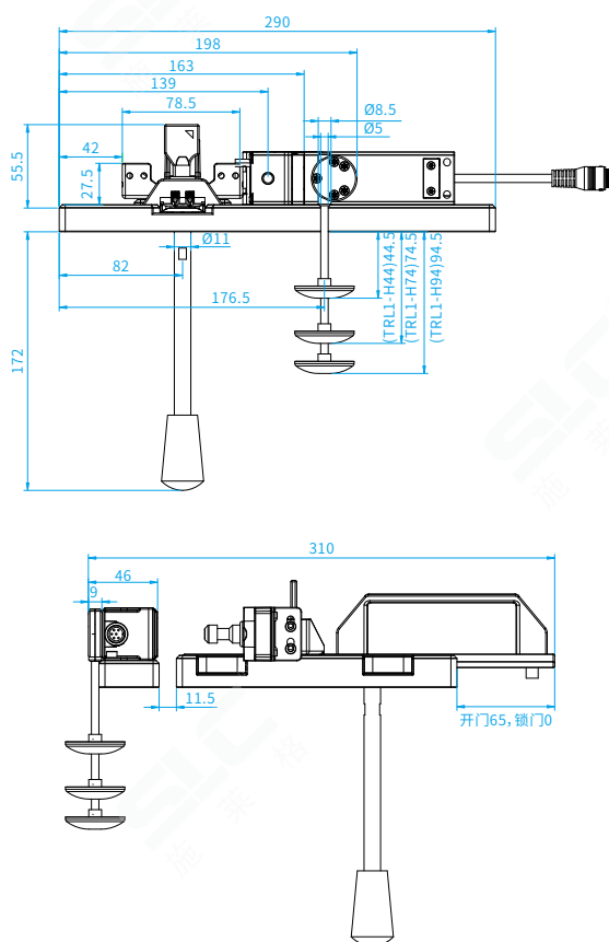
TRL1安全连锁(右开门)安装尺寸
