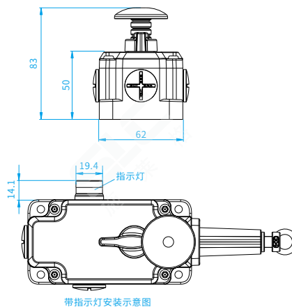
带指示灯安装示意图
