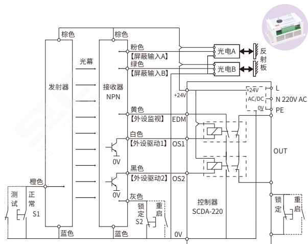
SLC-LP系列安全光栅（NPN）与控制器接线图
