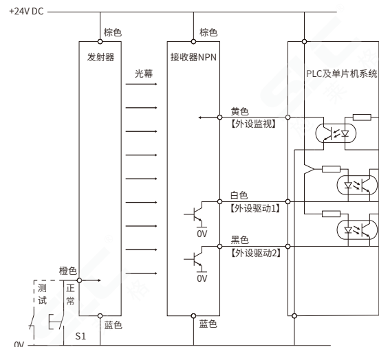
SLC系安全光栅（NPN）与PLC及单片机系统接线图
