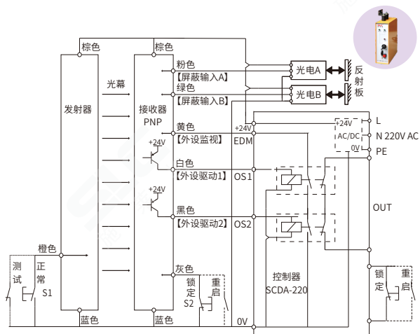
SLC-LP系列安全光栅（PNP）与控制器接线图
