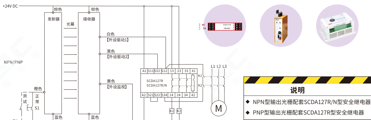
SLC系列安全光栅与安全模块接线图
