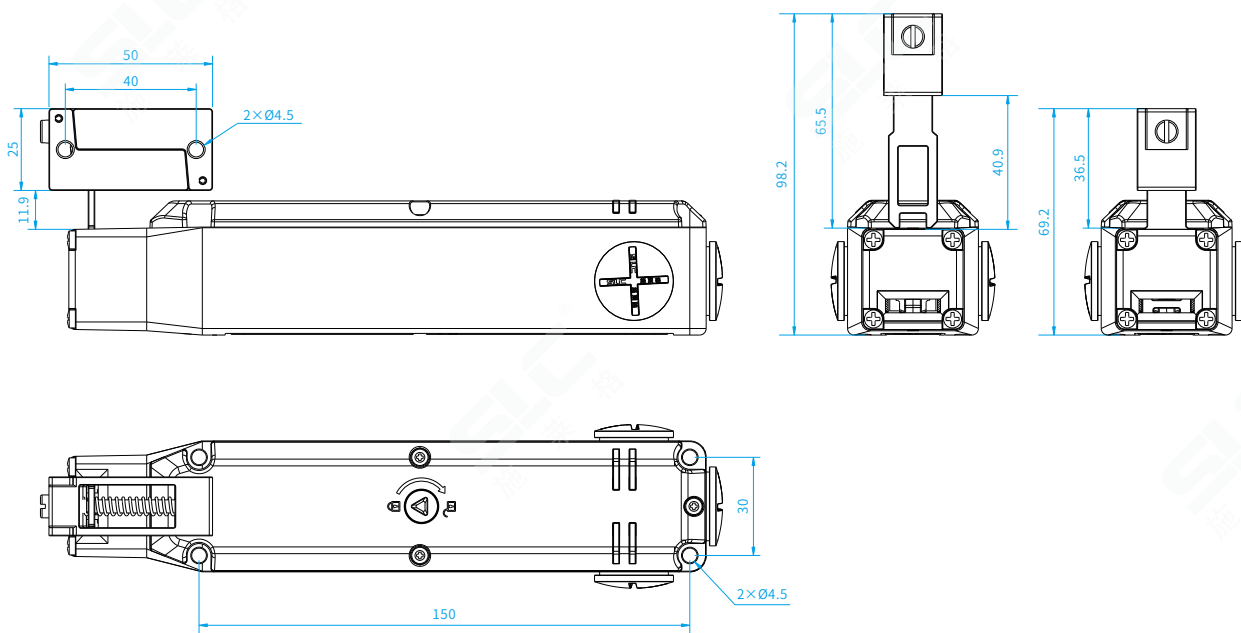
柔性钥匙从执行头正面插入
