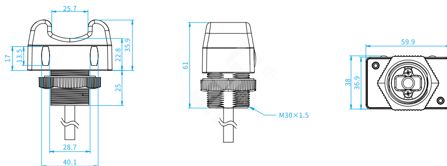
◆ TSB1无保护罩安装尺寸
