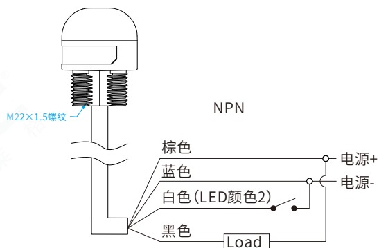
◆ SMLT30两色灯(功能2)接线示意图
