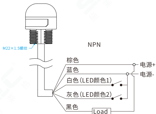
◆ SMLT30三色灯接线示意图
