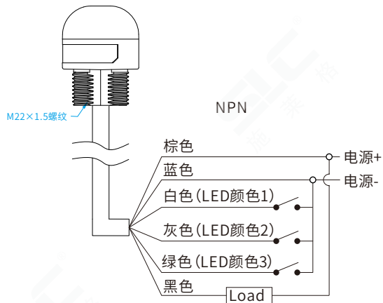
◆ SMLT30三色灯接线示意图
