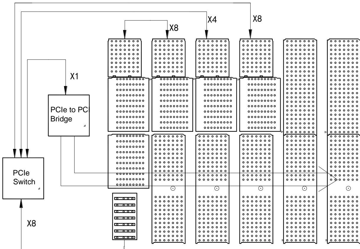
图 4 总线拓扑图
