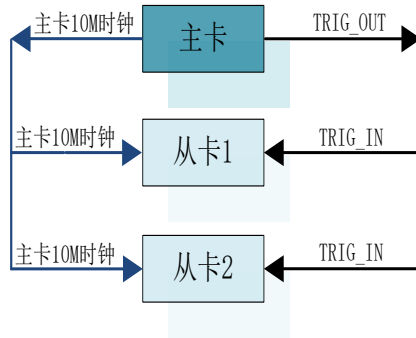
图 4-9-1 主从卡级联
