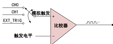
图5-3-2 模拟触发比较器
