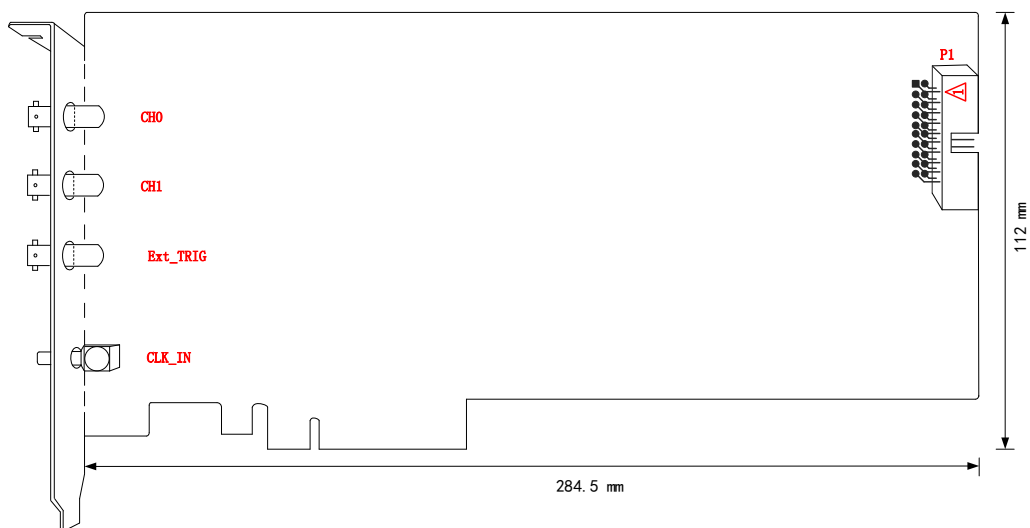
图 3-2-1 PCIe8910 板卡尺寸图
