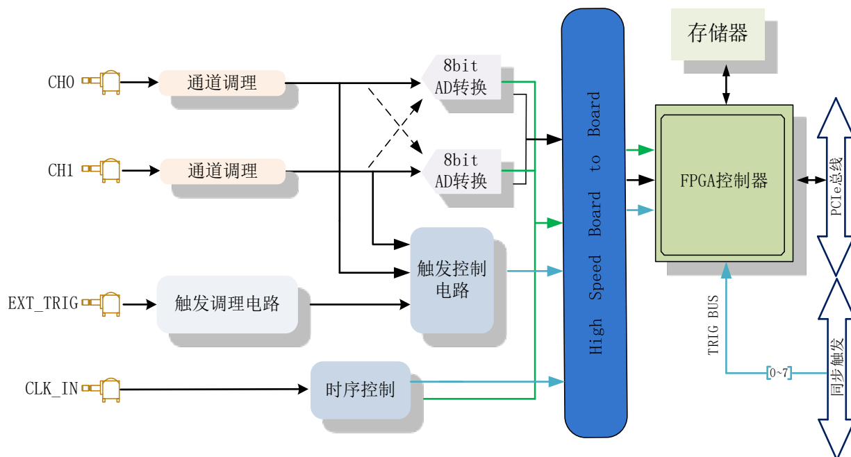
图 3-1-1 PCIe8910 系统框图
