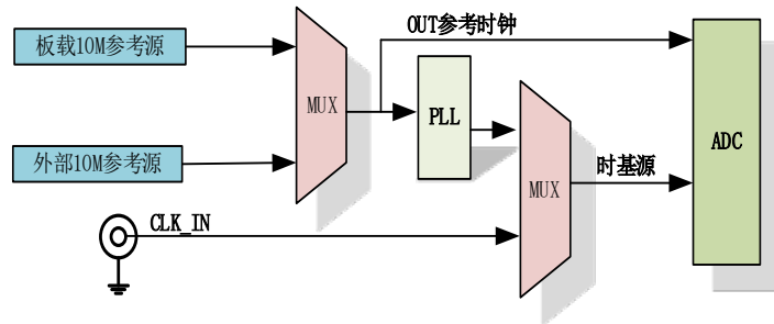
图 4-7-1 时基源框图
