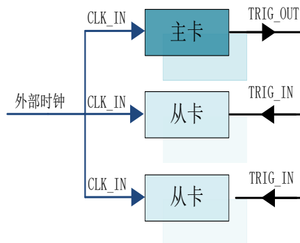
图 4-9-2 采用共同外时钟
