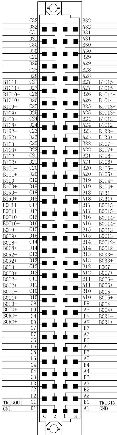
图 3-2-1 连接器引脚定义
