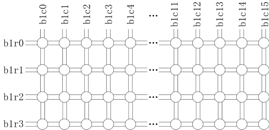
图 2-2-3 2 线双 4×16 矩阵 (配合 TB2601-D4_16)
