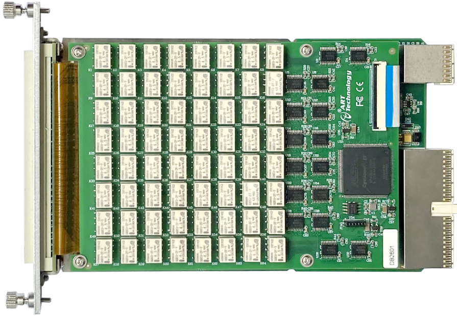
图 3-1-1 PXI2601 外形图
