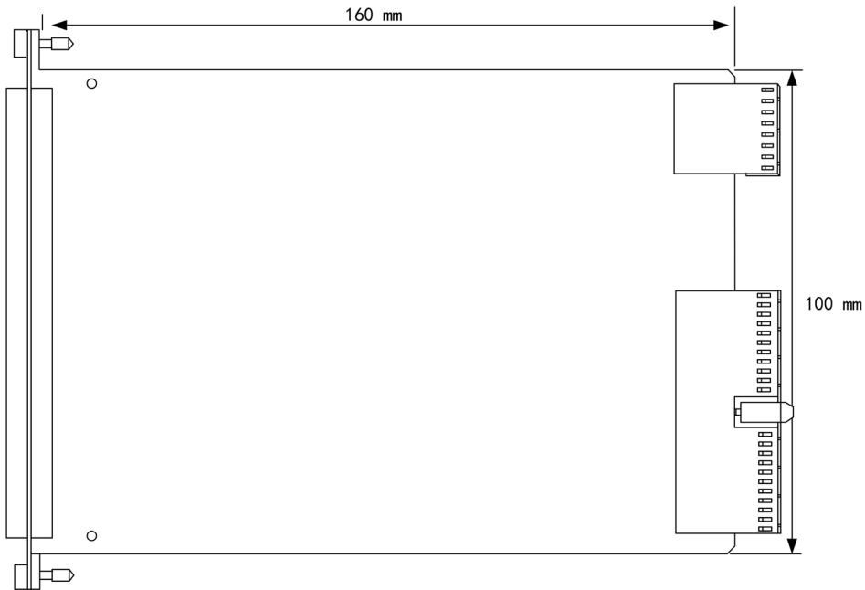
图 3-1-1 PXI2601 尺寸图
