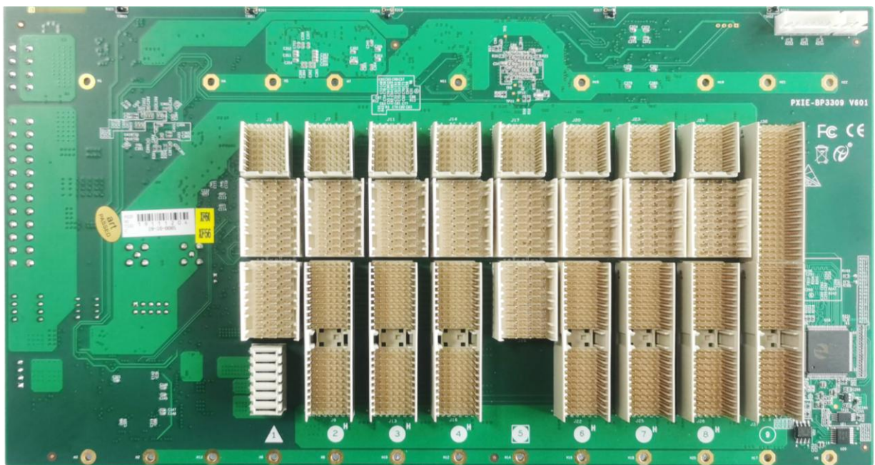
图 2-4 PXIEC-7309 背板
