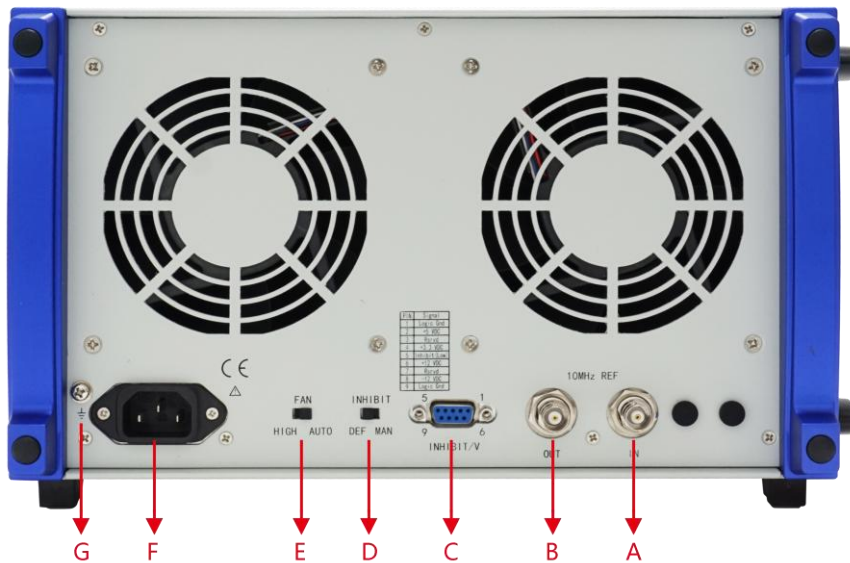
图 2-2: PXIeC-7309 后面板
