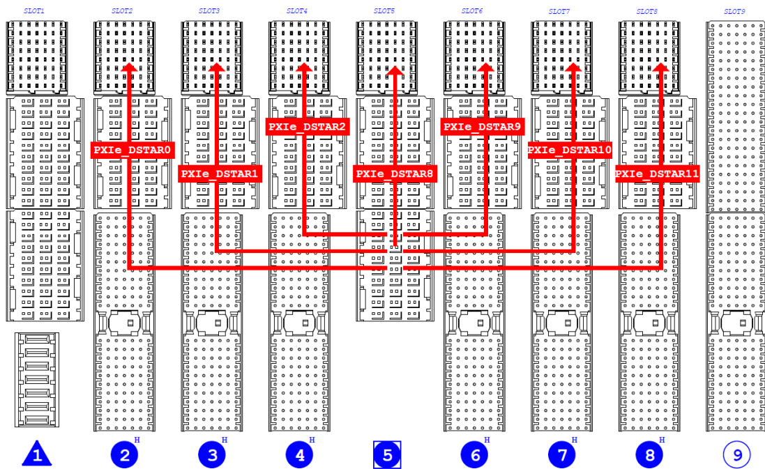
图 2-6 差分星形触发
