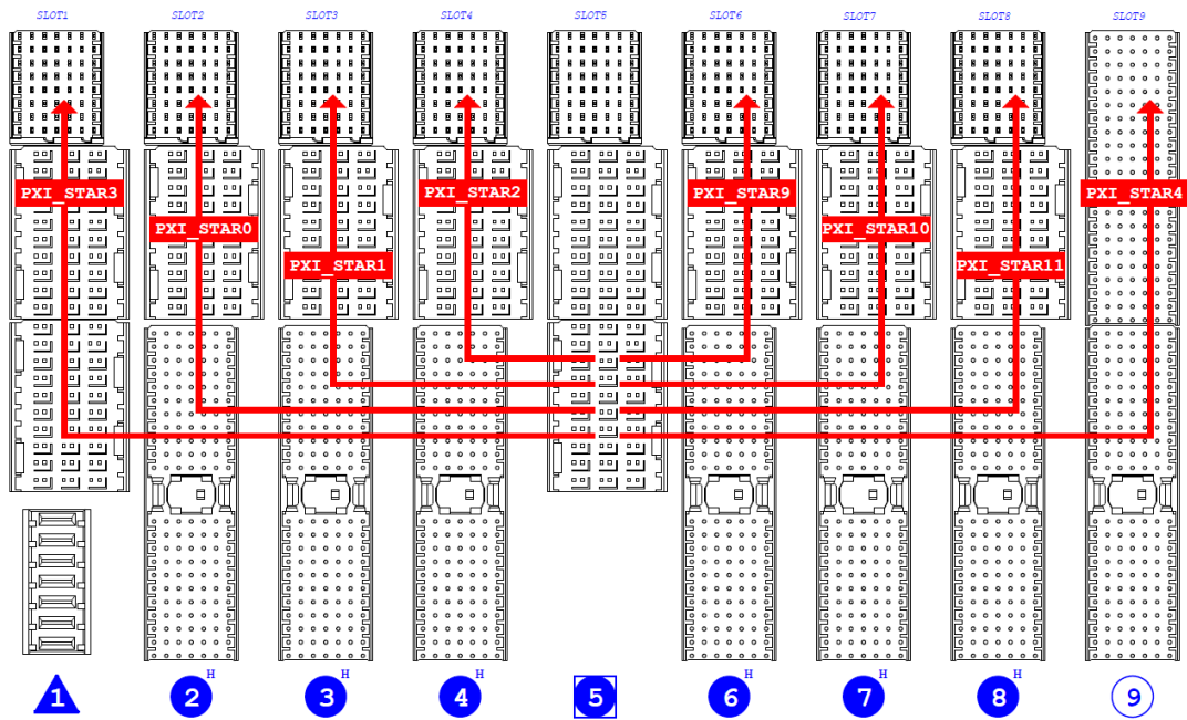
图 2-5 单端星形触发
