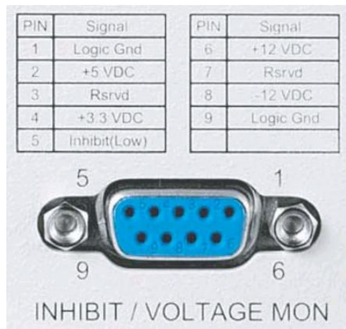
图 2-3 电源控制/电压监测接口
