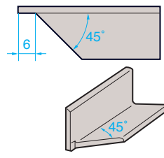
45° 角切槽刀/コーナノッチ
