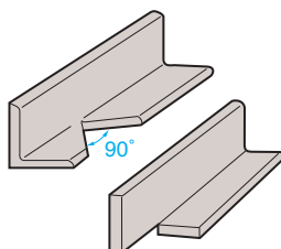
V型开槽刀/Vノッチ
