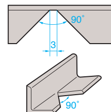
冲头切槽刀(特)/ポンチノッチ特
