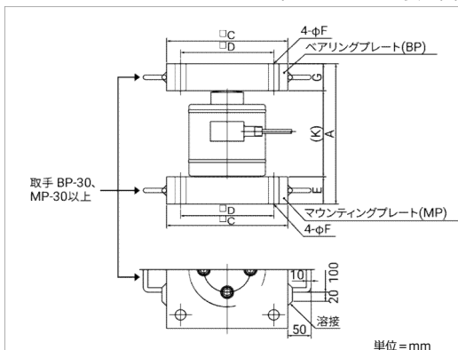
ベアリングプレート・マウンティングプレート装着図
