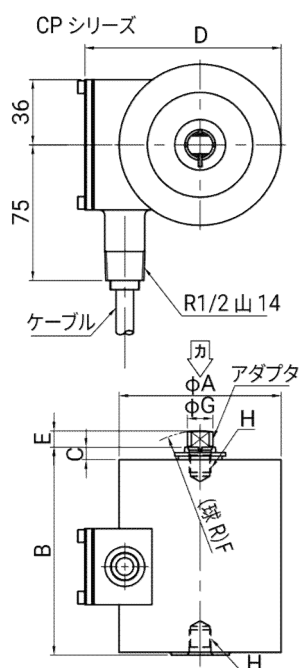
外形寸法図
