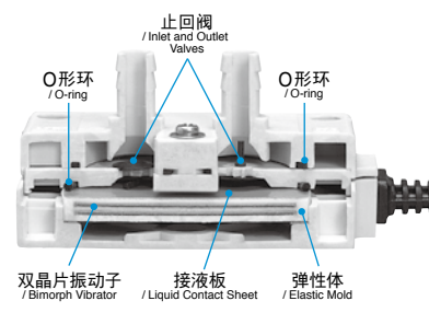
截面图 / Cross section
