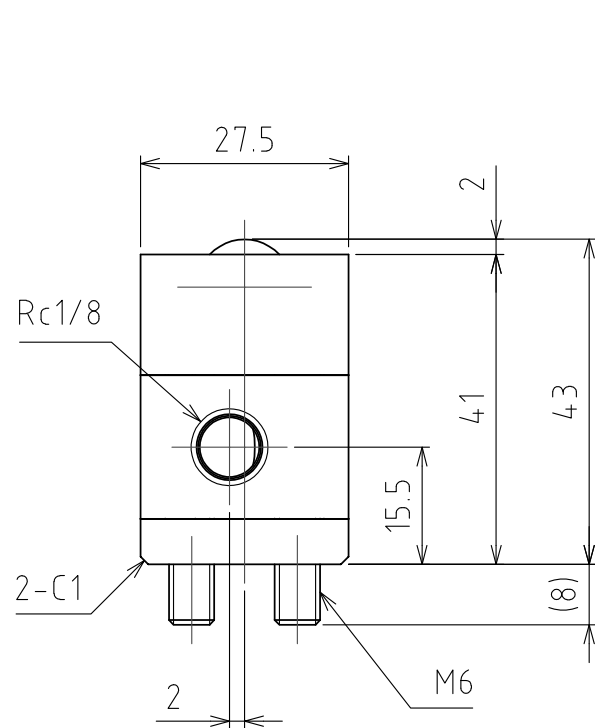
A矢視図
