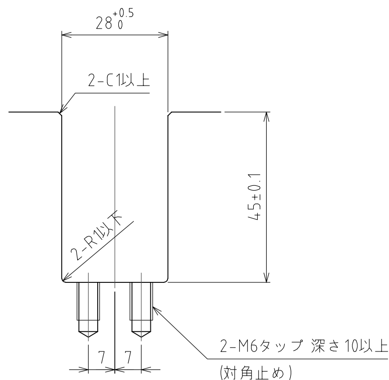
推奨溝寸法
