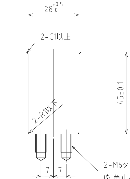
推奨溝寸法
