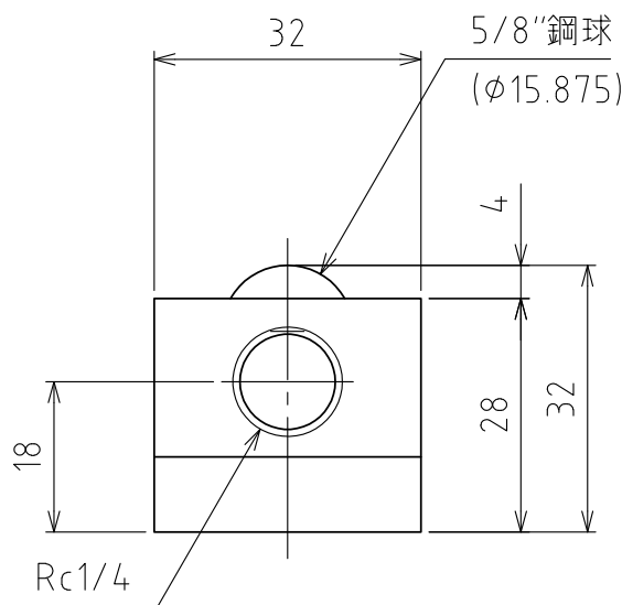
A矢視図
