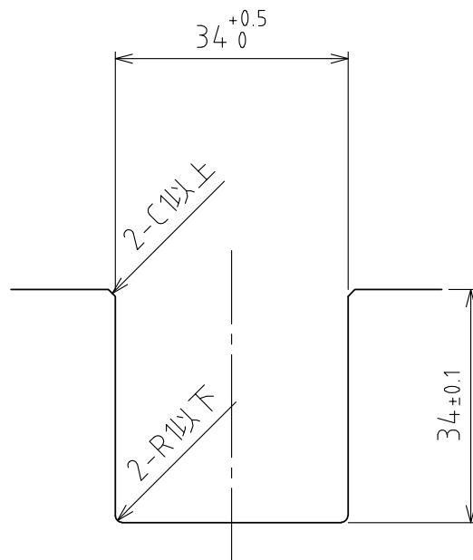
推奨溝寸法
