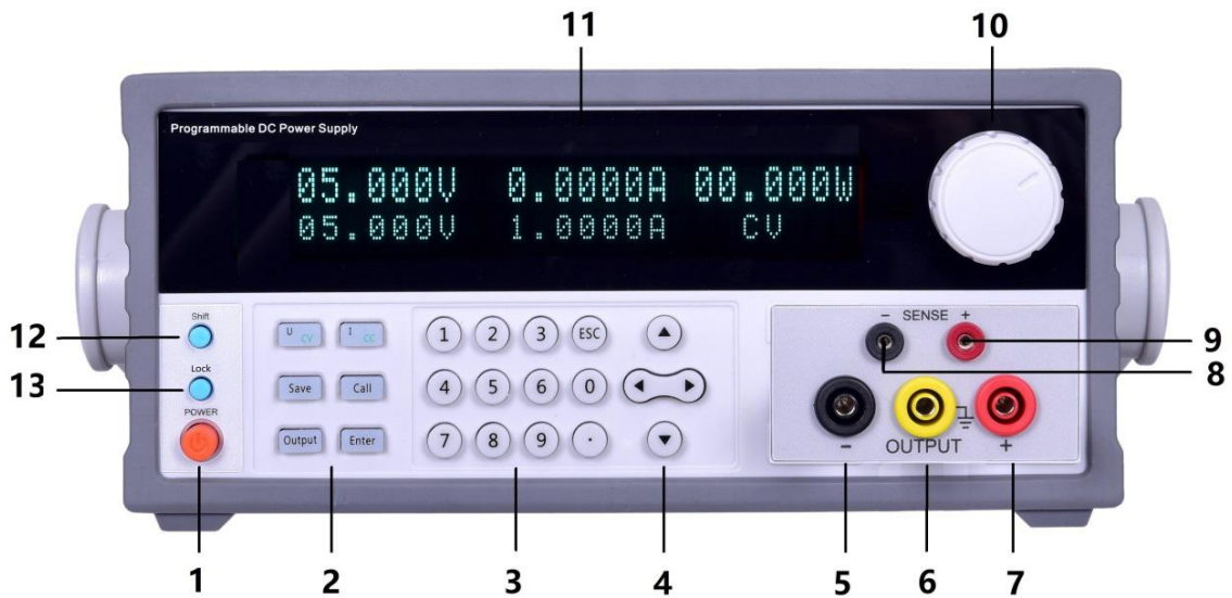
前面板图
