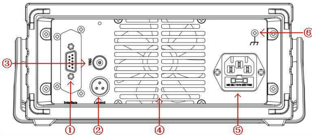
后面板图
