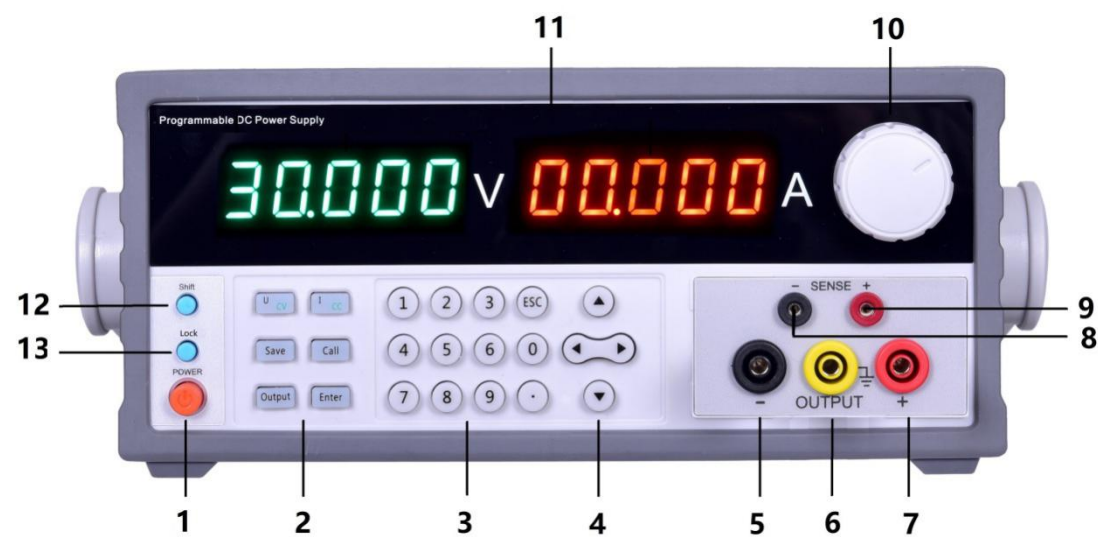
前面板图
