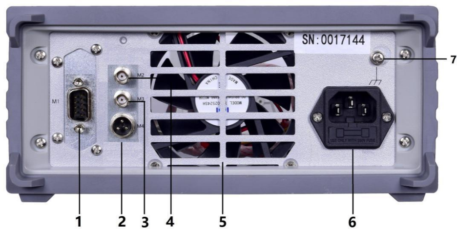
后面板图
