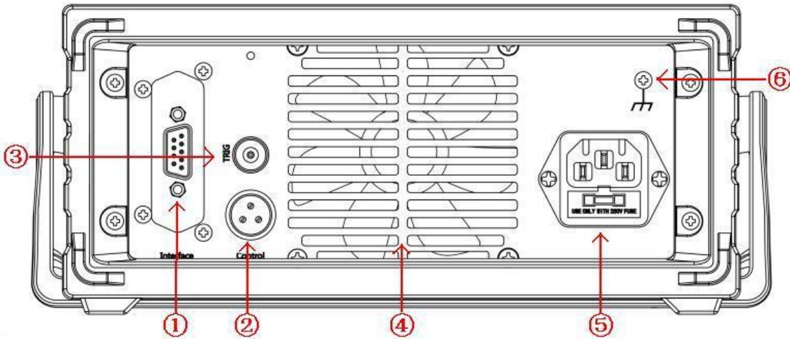
后面板图
