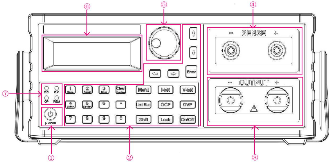
前面板图
