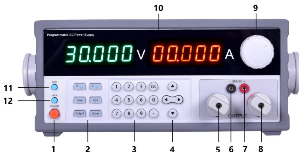
前面板图
