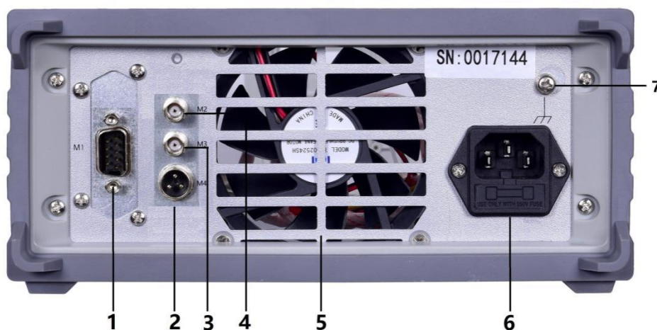
后面板图
