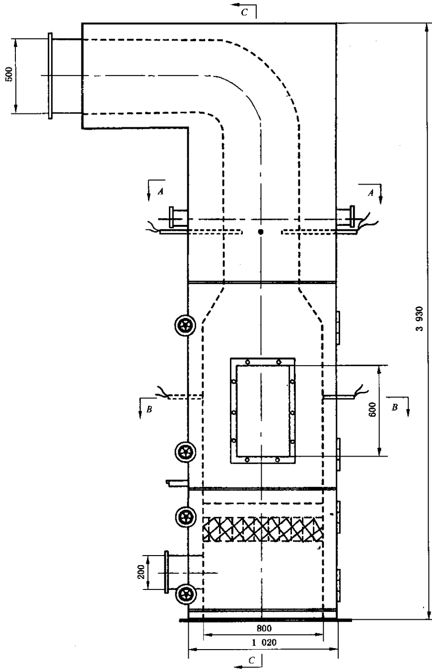
图 1 燃烧竖炉
