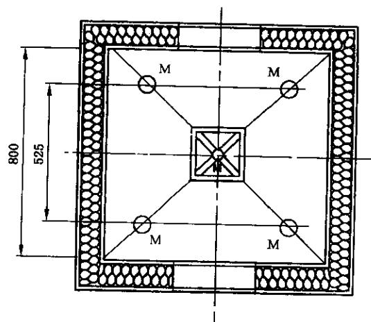
图 5 空气均匀性试验测点位置
