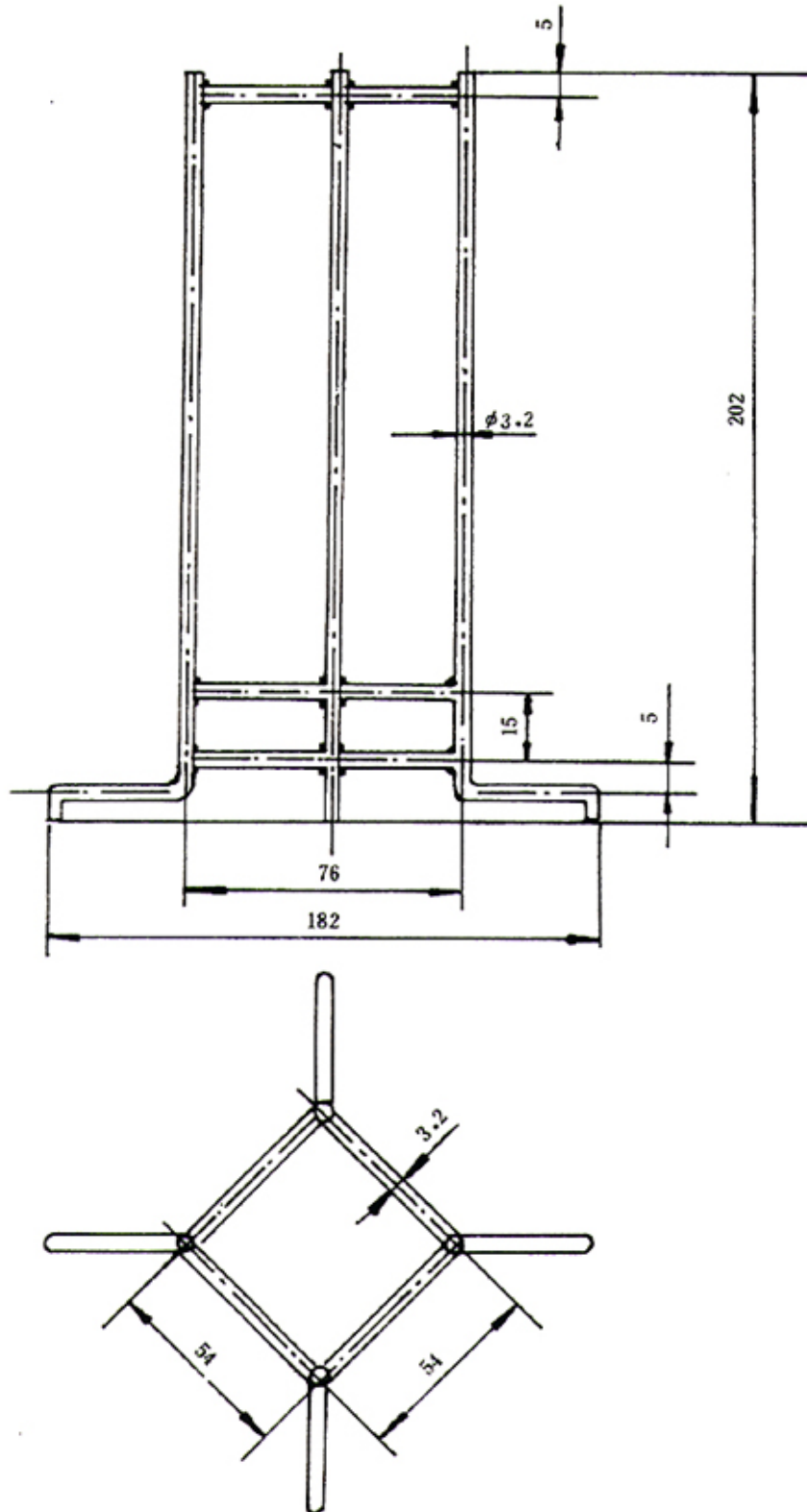
图1 试件支承架
