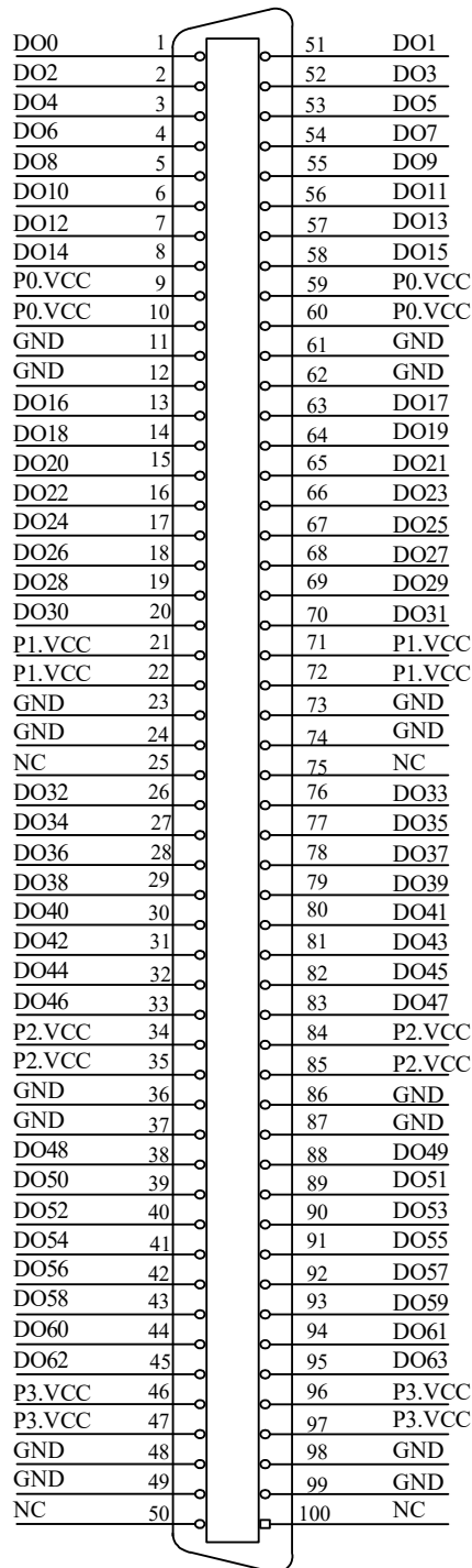
图 3-3-2 PCIe2332A 接口定义
