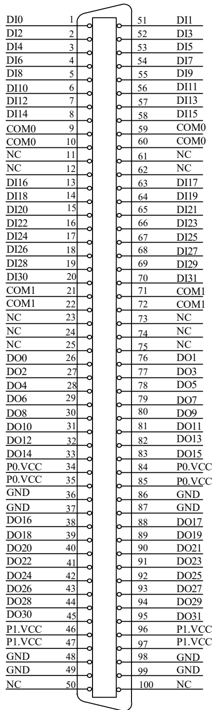
图 3-3-1 PCIe2330A 接口定义
